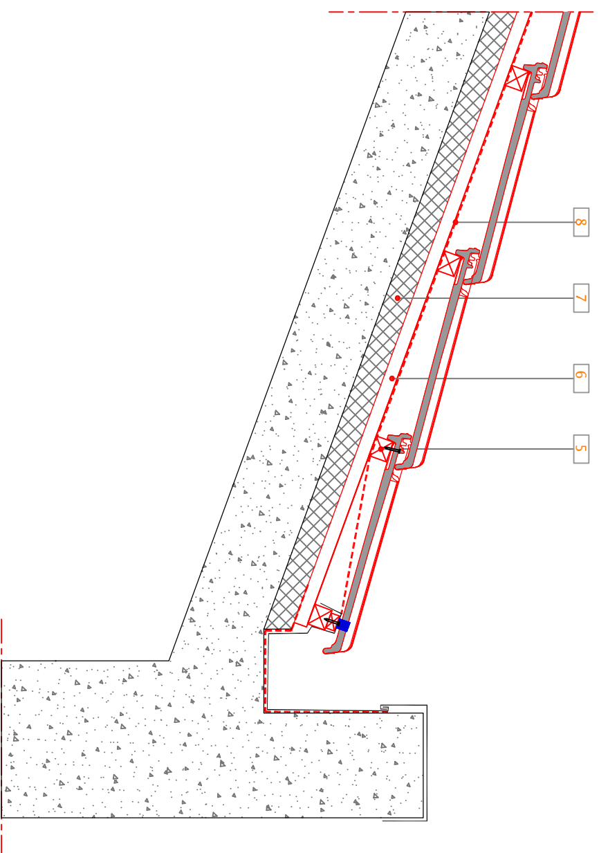
261 Corte vertical transversal - Pormenor ripado + contra-ripado
