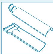
Beirado Bica e Capa 0,60 Underlover eave tiles 0,60
