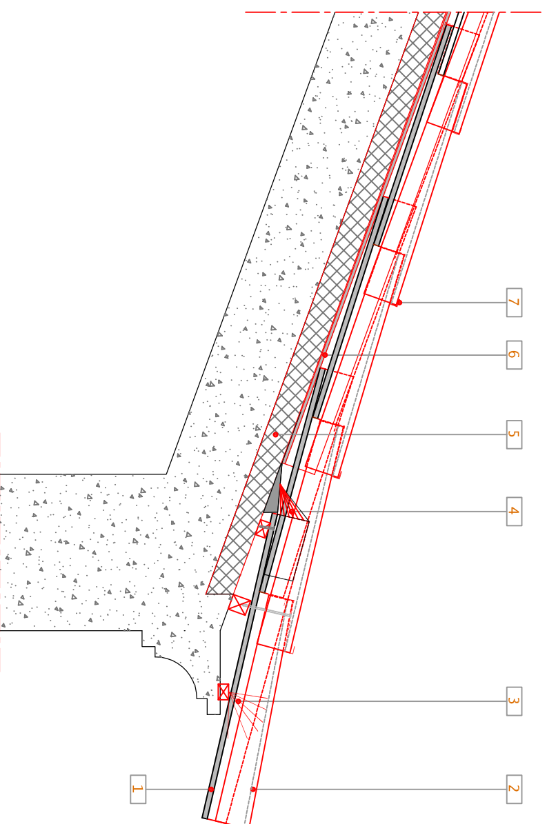
332 Corte vertical transversal - Pormenor com subtelha UM placa 190
