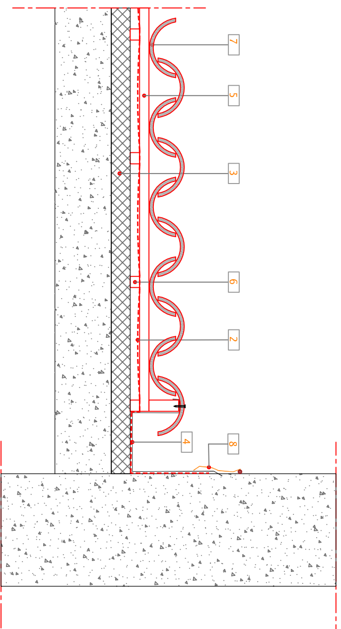
381 Corte vertical [longitudinal] - Pormenor ripado + contra-ripado
